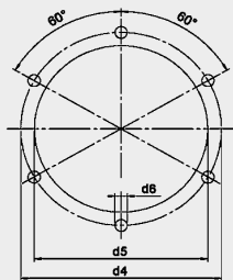
Interface to DIN 24557/Pt 2
